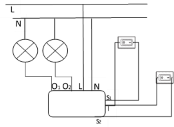
דיאגרמת חיבור בקר תאורה חכם או בקר תריס חכם
