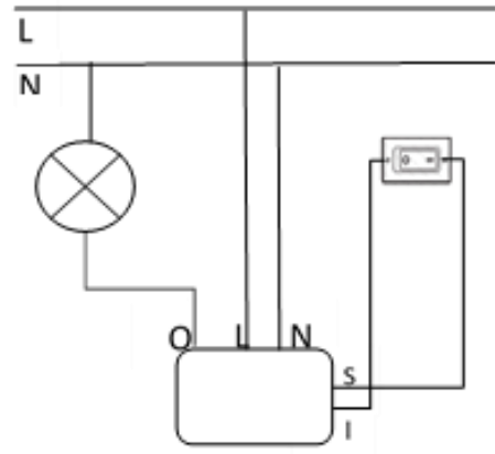
דיאגרמת חיבור בקר תאורה חכם או בקר שקע חכם
